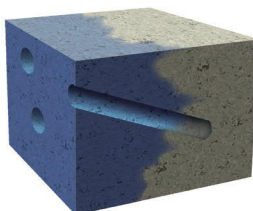
1) 在墙壁上按照40-80°的角度钻孔，深度约为3/4墙厚。
