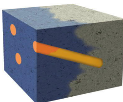
2) 使用 PENETRON 澎内传防水涂料（PNC401）浆料灌满钻洞。使用 PENECRETE MORTAR 澎内传修补砂浆（PNC302）封闭洞口。
