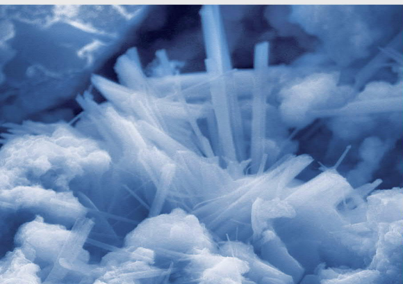
PENETRON 澎内传中的活性成分催化混凝土中的水泥水化产物反应后形成的结晶体照片，这些晶体结构可填充和封堵宽度达 0.4mm 的裂缝、孔洞和空隙。（放大倍数5000x）
